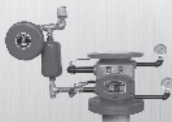
罐式报警阀
